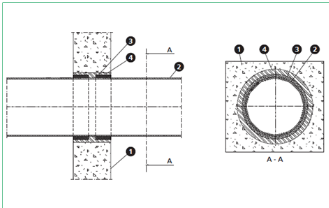
2. ábra: Ø > 110 mm-es műanyag cső átvezetése tömör falon keresztül
